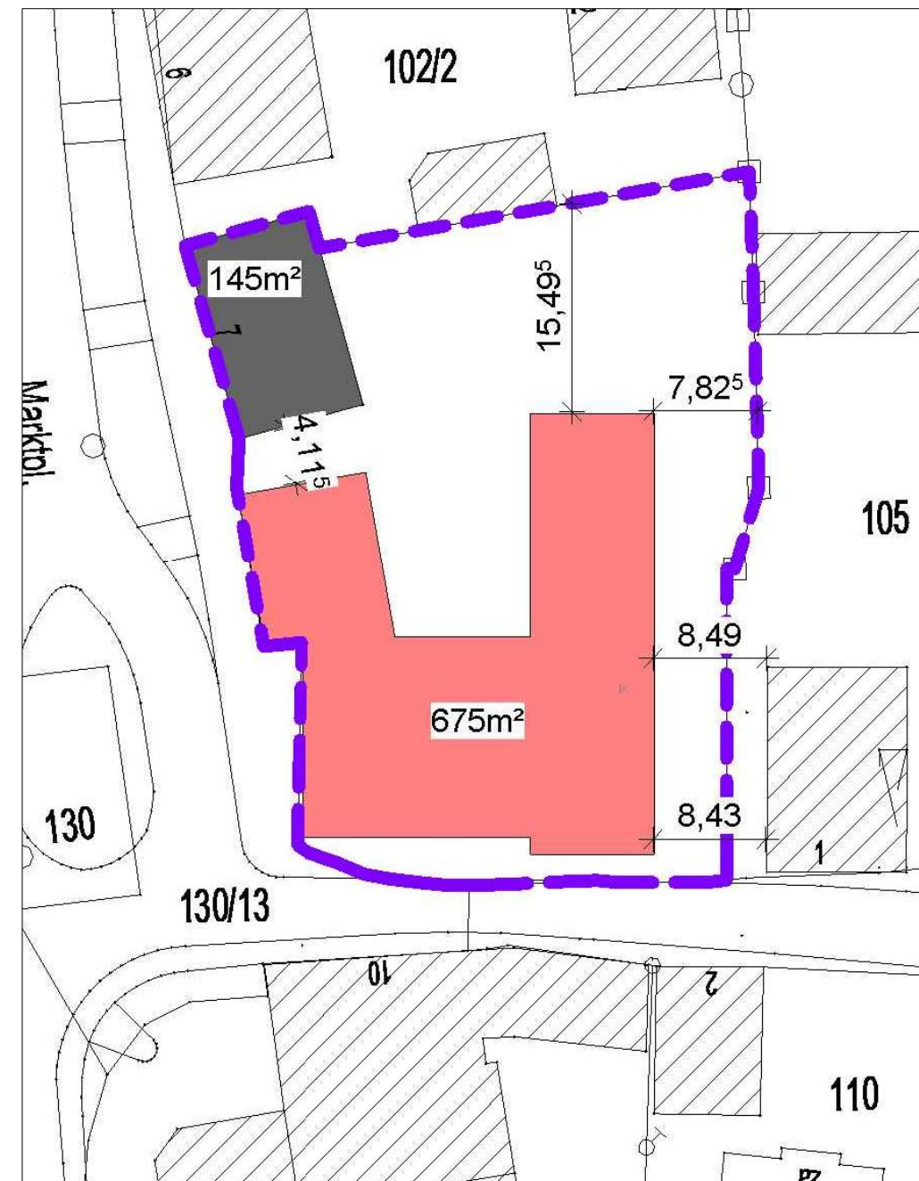
Bebauung Neubau
